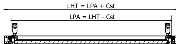
A-A ( 1:10 )
