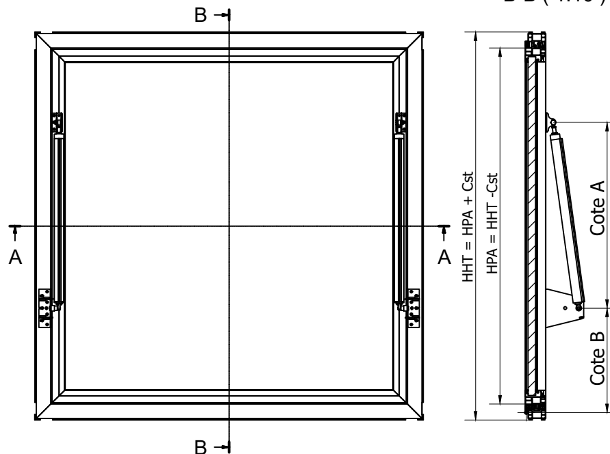
B-B ( 1:10 )
